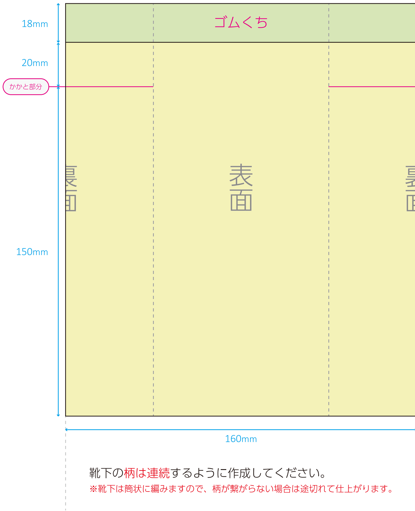
展開図
