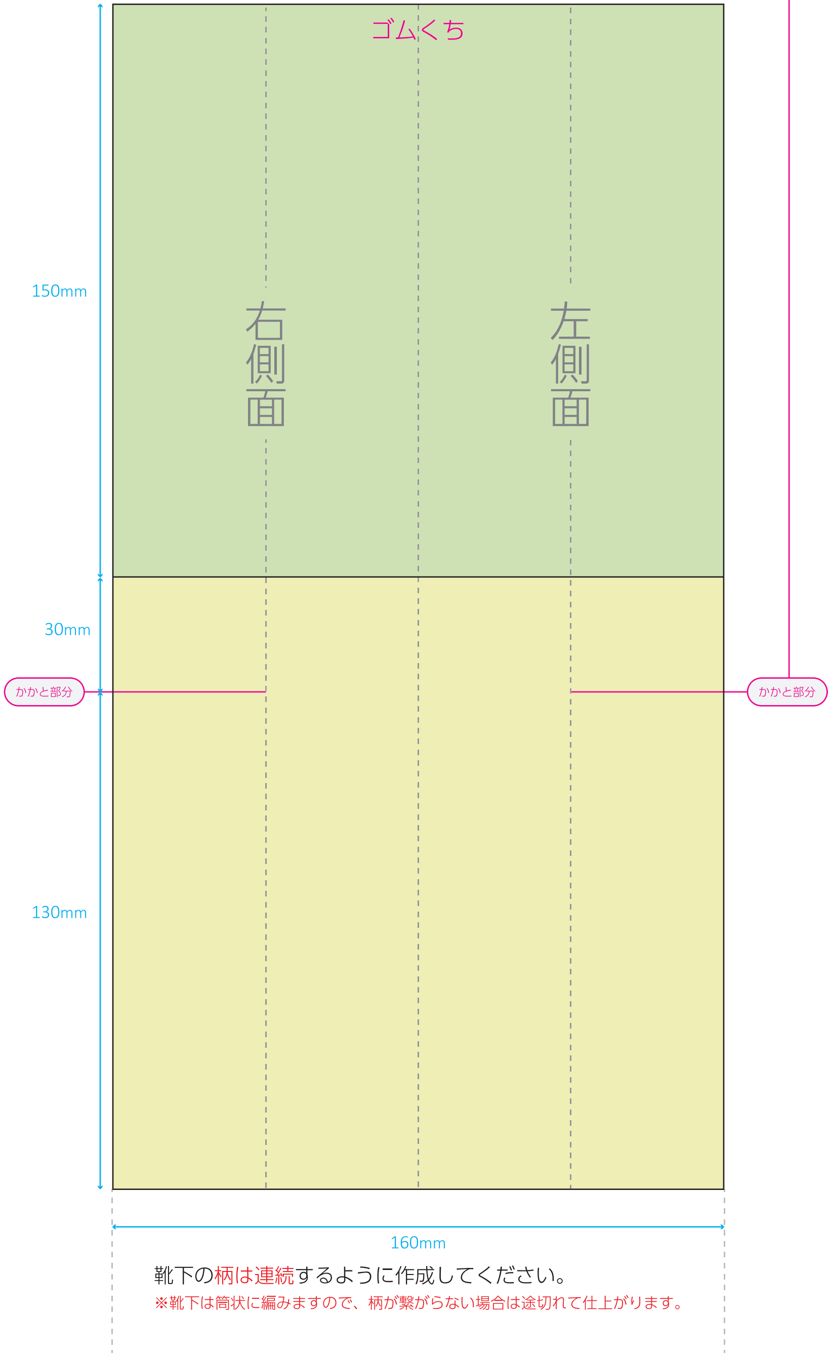
展開図
